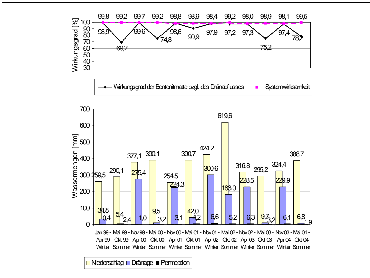
Bild 2: Lysimeter 3 – Auswirkungen von Sommer- und Winterzyklen auf die Dichtungswirkung einer einschichtigen Standard-Bentofix-Bentonitmatte
