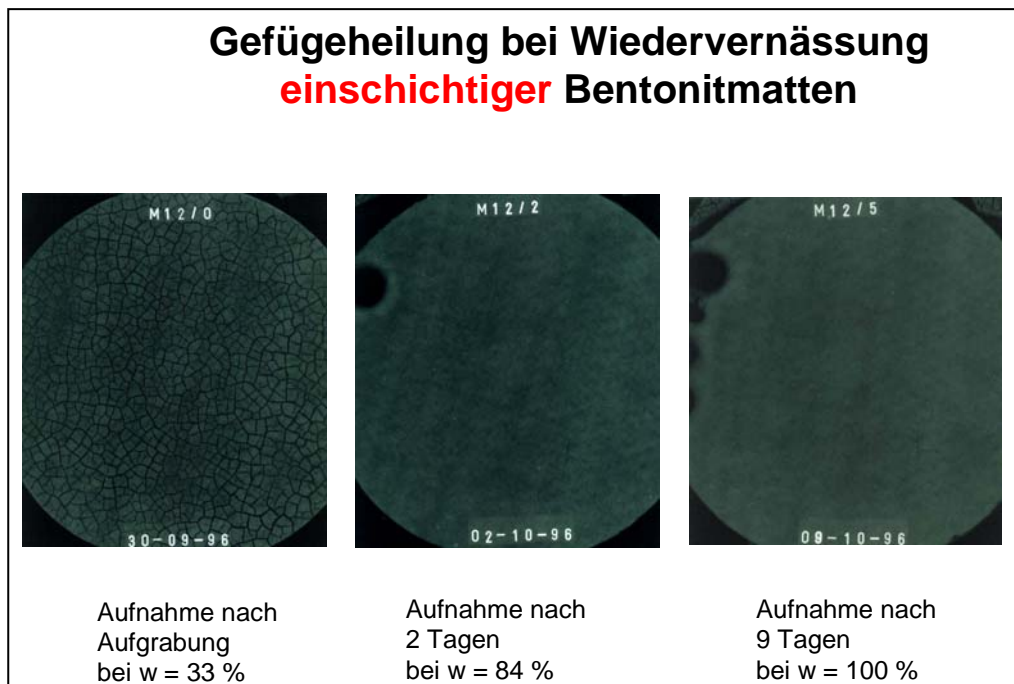
Bild 1: Gefügeheilung bei Wiedervernässung einschichtiger Bentonitmatten
