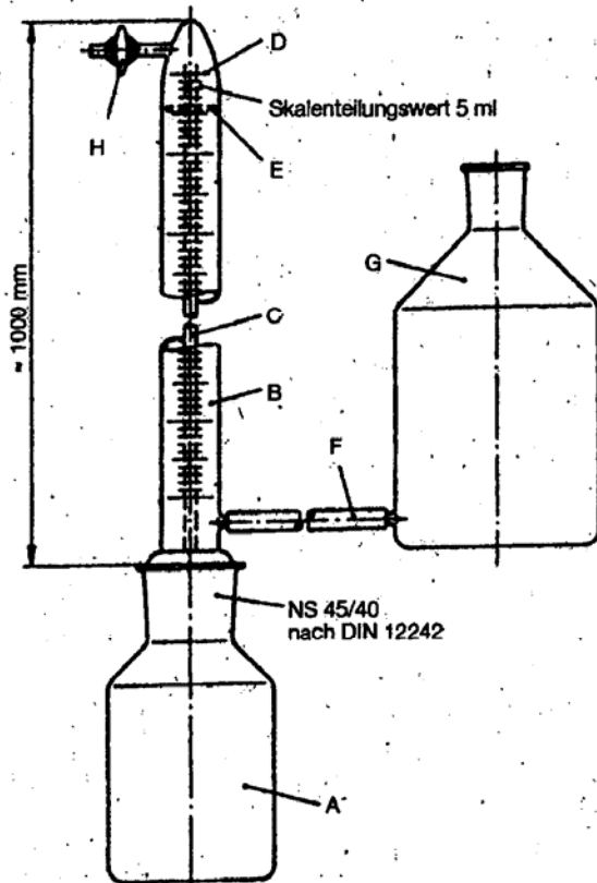
Bild 2: Versuchsanordnung zur Bestimmung des Faulverhaltens von Schlamm [DIN 38414 Teil 8, Seite 6]
